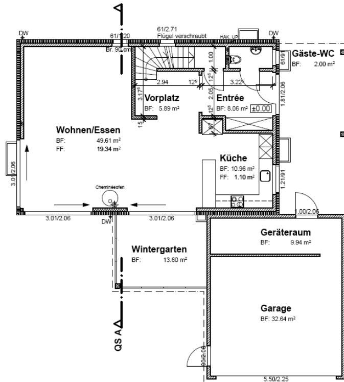
Erdgeschoss
