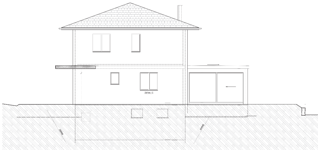
Nordwestfassade
