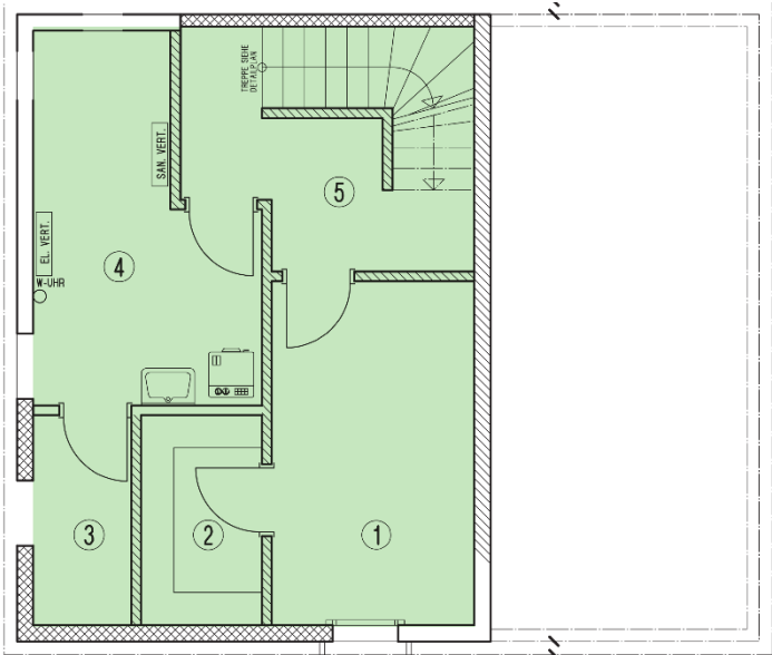
Untergeschoss
