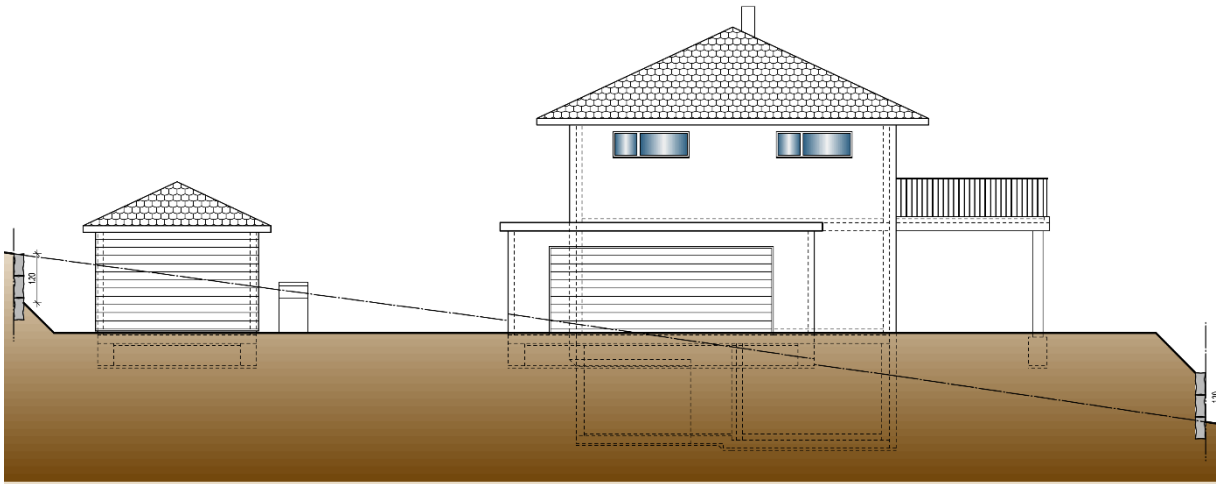
Westfassade
