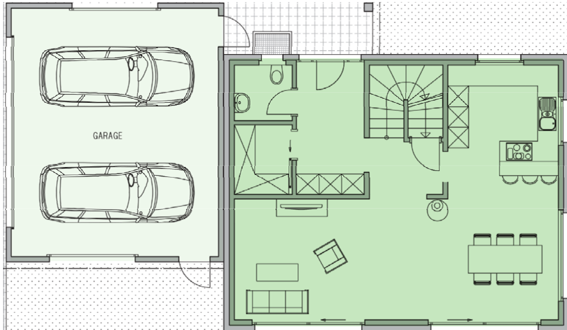
Erdgeschoss
