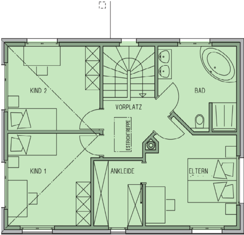
Dachgeschoss
