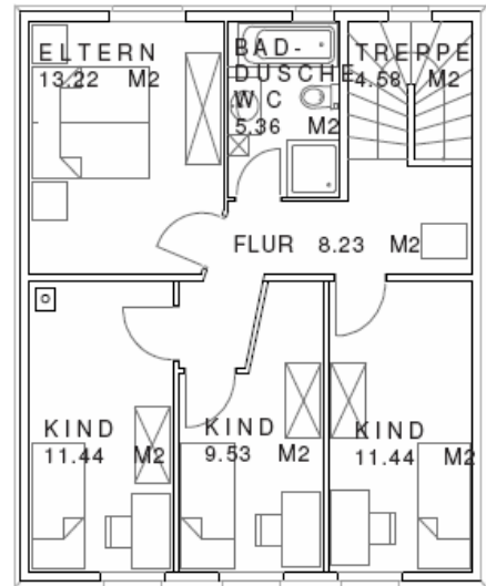
Obergeschoss 8.21 x 9.41m
