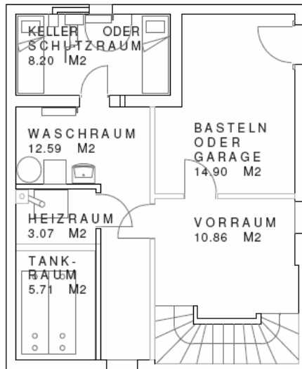
Kellergeschoss 7.89 x 9.09m
