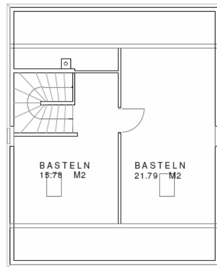
Dachgeschoss 8.21 x 9.41m
